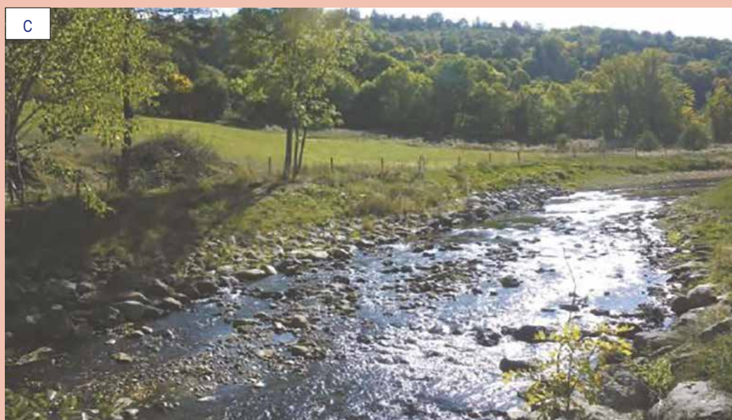
Figura 30 – Rimozione di una briglia (visibile in A) sul torrente Alagnon, un affluente dell'Allier nel bacino della Loira (Francia).
