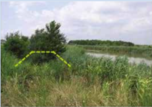
Figura 6 – Esempio di arretramento arginale sul fiume Zero (Provincia di Venezia).
