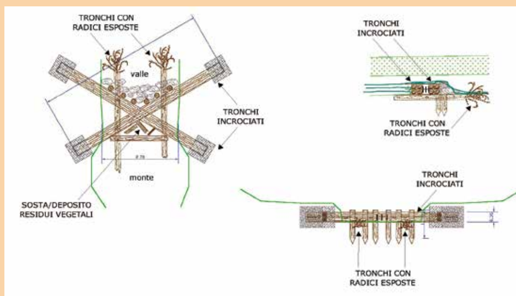
Figura 37 - Schema progettuale di massima dell'intervento di costruzione di strutture trasversali atte ad aumentare la capacità di sedimentazione e rialzare il livello dell'alveo. Immagine: Consorzio di Bonifica dell'Emilia Centrale (RE).
