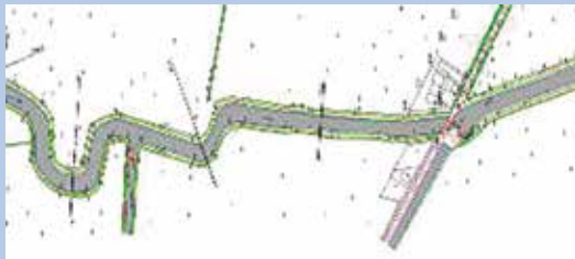
Figura 14 – Esempio di creazione di una piana inondabile sul torrente Bevano (loc. San Zaccaria in Comune di Ravenna)
