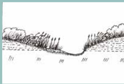
Figura 49 – Schema progettuale di massima dell'intervento Disegni Regione Emilia-Romagna: Massimo Milandri
